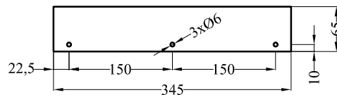
blacha 3x65x345
